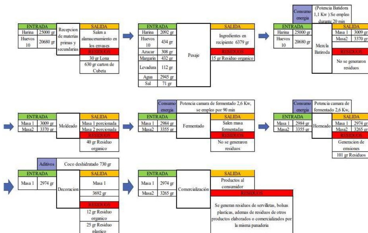
Figura 10. Eco balance de un día de producción en la panadería. Elaborado por (Mahecha Valderrama, 2020)
